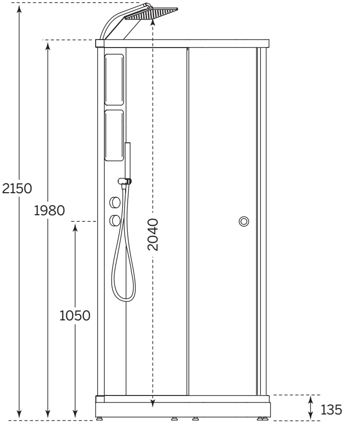
Infälld blandare / Recessed mixer / Innfelt blande­batteri
