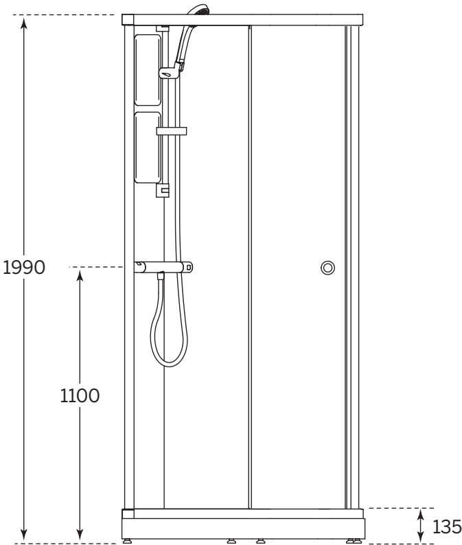
Standard & Standard blandare /mixer /blandebatteri
